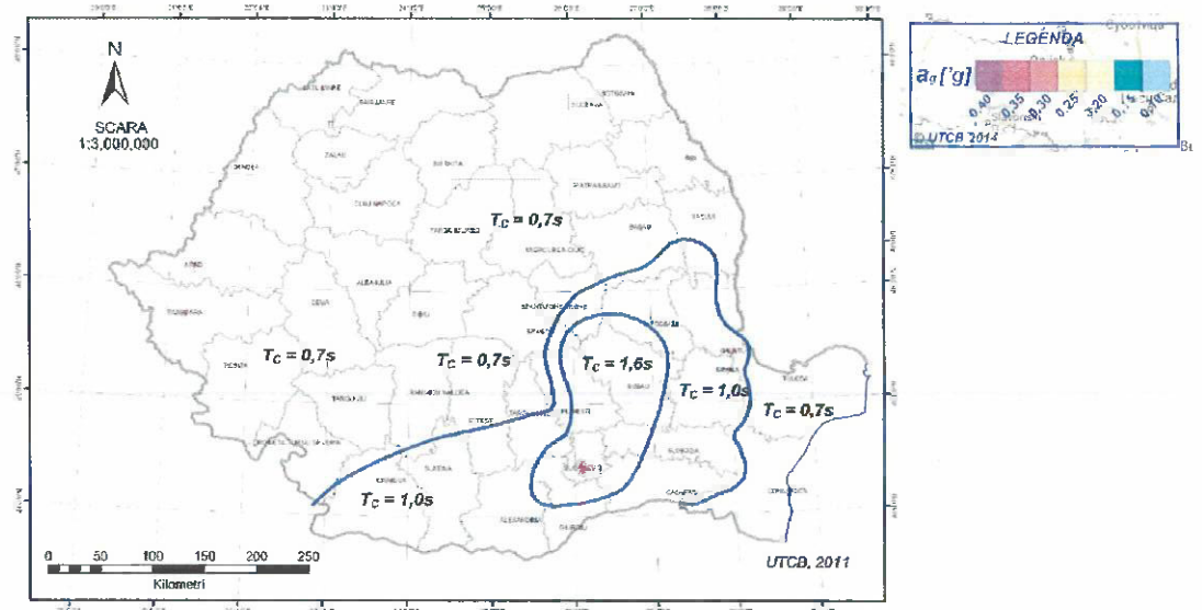
Fig. 3 - Perioada de control (colț) a spectrului de răspuns T_c = 1.6 sec, P 100 / 1 – 2013
