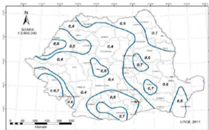
Figura 2.1 Zonarea valorilor de referință ale presiunii dinamice a vântului, q_0 , în kPa, având IMR = 50 ani
