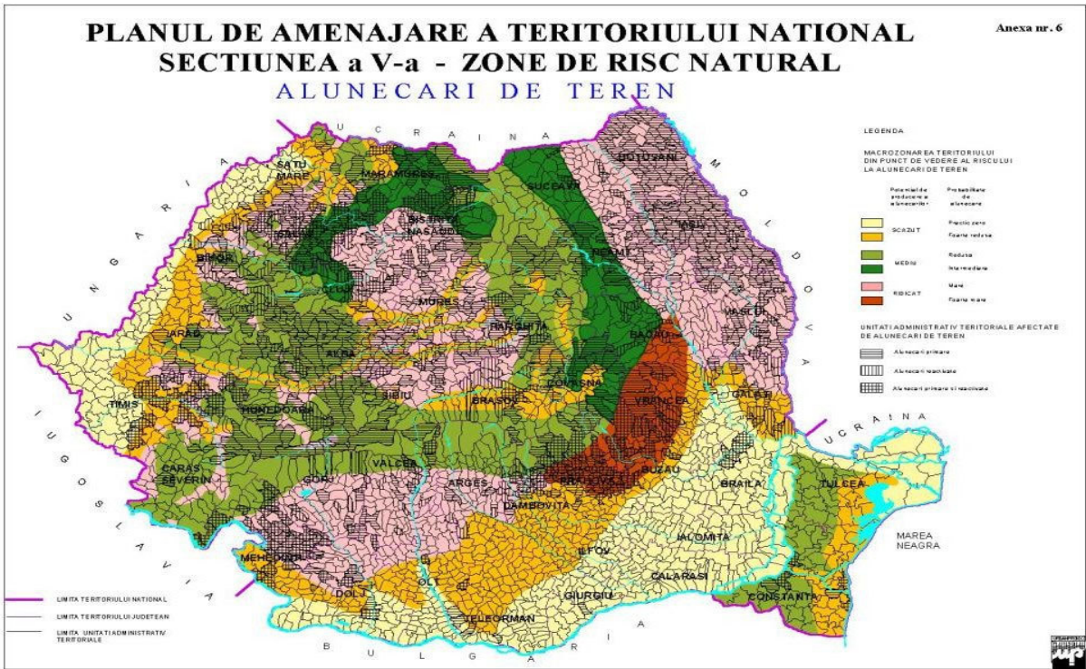
Figura 3-6 Zonarea teritoriului functie de potentialul producerii alunecărilor de teren.
