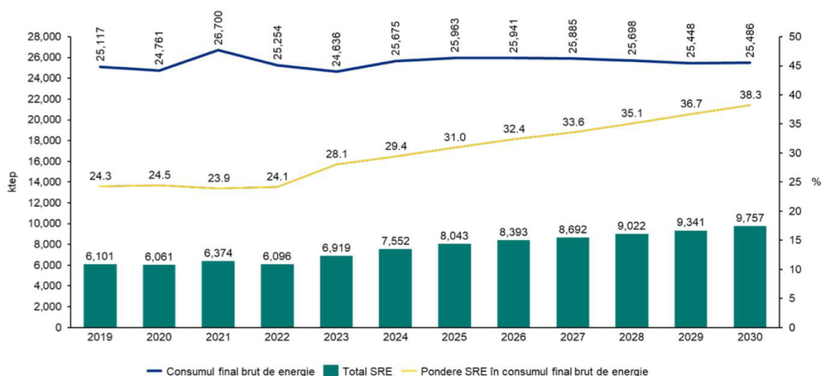
Figura 2.8 – Sinteza evoluției ponderii de energie, pe sursa primară, în România, în perioada 2019 – 2030, conform (României, Planul Național Integrat în domeniul Energiei și Schimbărilor Climatice 2021 - 2030, 2021).
