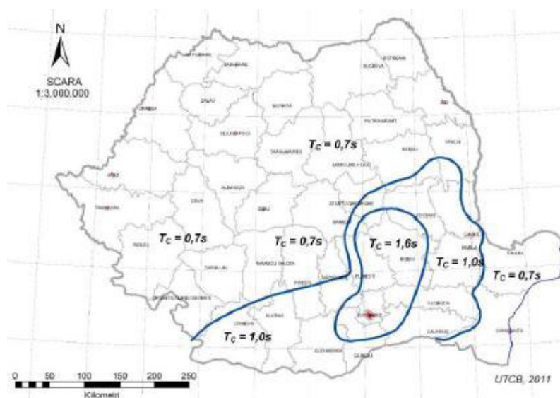
Figură 5 - Zonarea teritoriului României în termeni de perioada de control (colț), T_c a spectrului de răspuns
