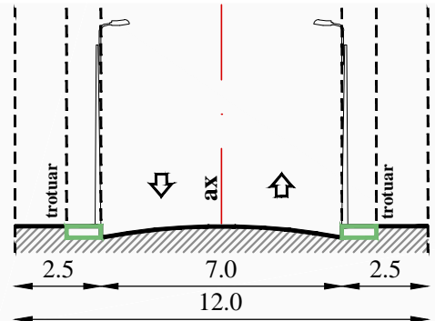
Profil existent si mentinut str. Margelelor sc 1:200
